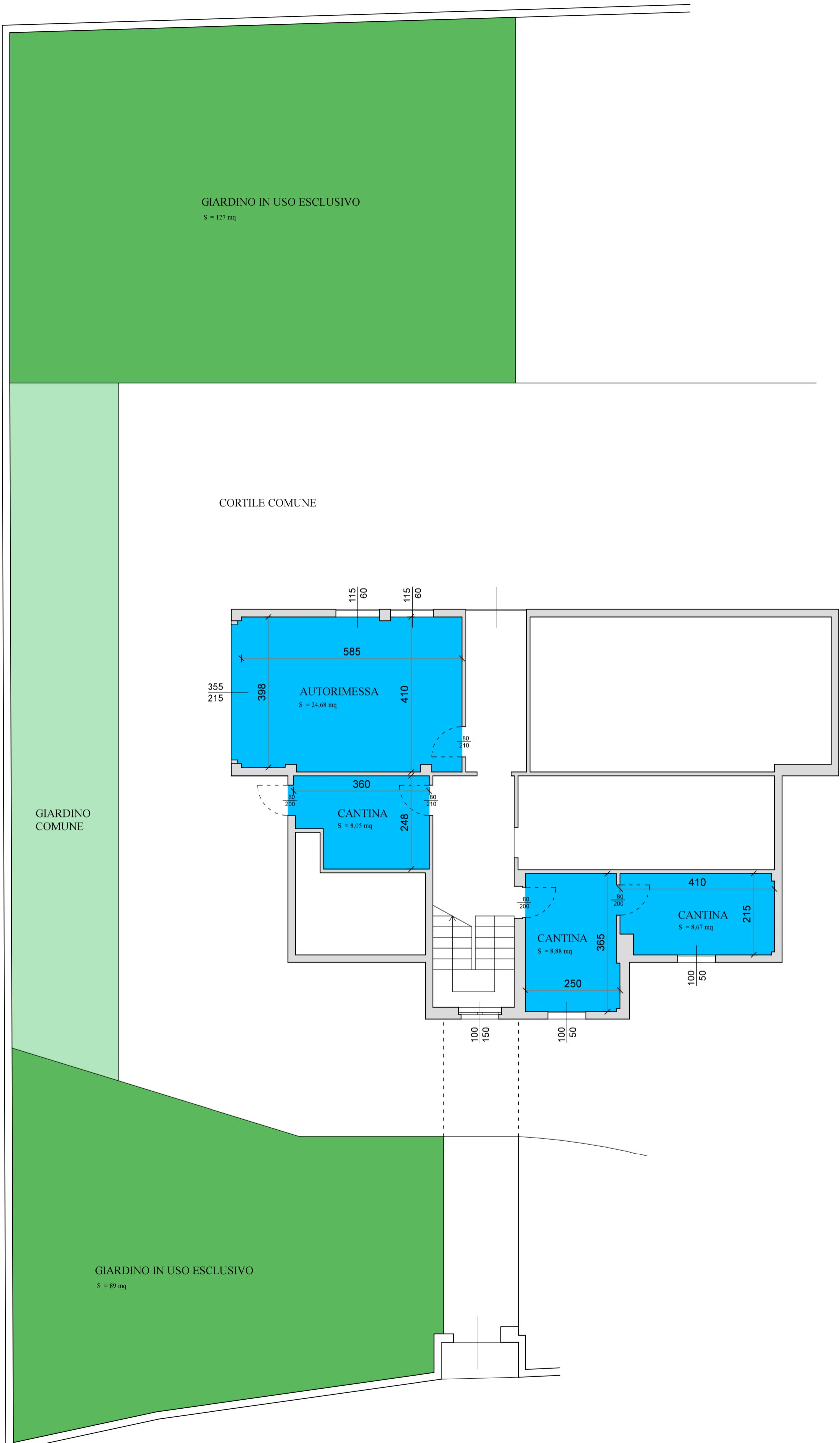
Pianta Piano Seminterrato H. 260 cm
